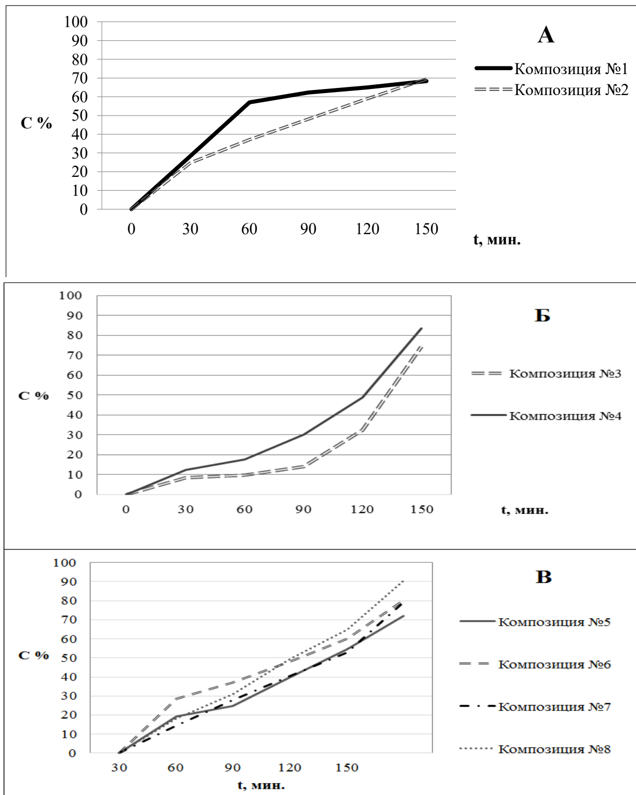
Рис. 1. Динамика высвобождения фурацилина из стоматологических гелей: А – на основе МЦ; Б – на основе желатине; В – на основе ПВХ
