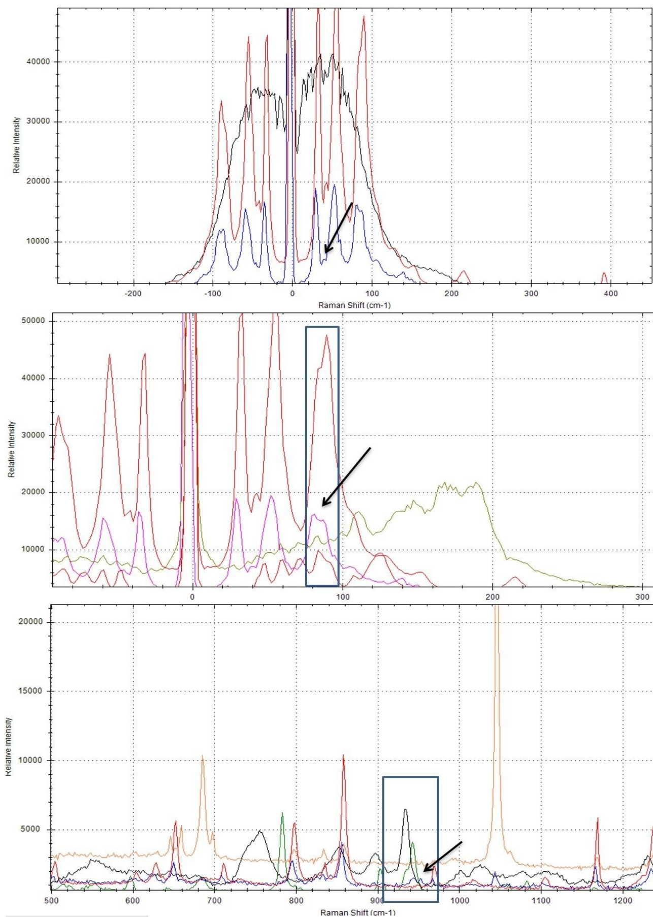
Рис. 5. Спектр комбинационного рассеяния МС 2.5: парацетамол, карбонат натрия, гидрокарбонат натрия, повидон и лимонная кислота
